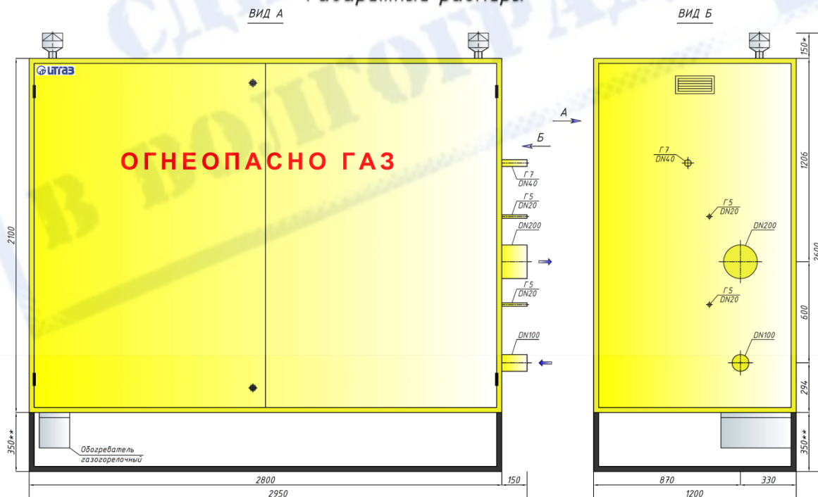
Габаритные размеры
